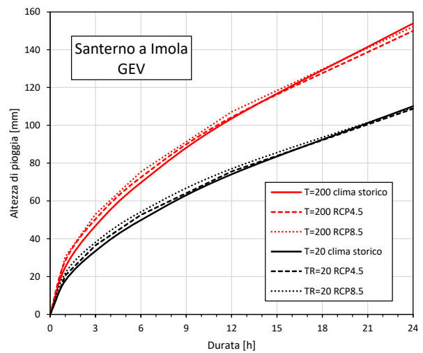
Figura 143 - Confronto tra le curve di possibilità climatica di T=20 e T=200 anni nel caso di clima storico e quelle del periodo 2041-2070 secondo le proiezioni di pioggia degli scenari RCP4.5 e RCP8.5, per il bacino del Santerno chiuso a Imola; a sx modello probabilistico di Gumbel, a destra modello probabilistico GEV.
