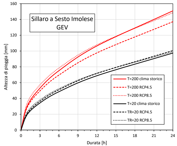
Figura 142 - Confronto tra le curve di possibilità climatica di T=20 e T=200 anni nel caso di clima storico e quelle del periodo 2041-2070 secondo le proiezioni di pioggia degli scenari RCP4.5 e RCP8.5, per il bacino del Sillaro chiuso a Sesto Imolese; a sx modello probabilistico di Gumbel, a destra modello probabilistico GEV.
