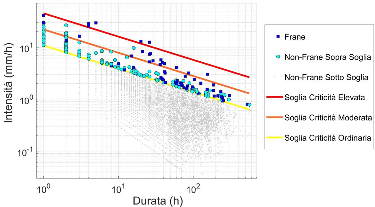
Figura 106 – Esempio di calibrazione su un periodo di 10 anni di un sistema di soglie pluviometriche a criticità crescente, definito considerando sia eventi franosi che non franosi.
